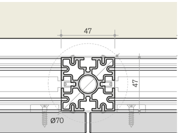
C. sezione orizzontale horizontal section
