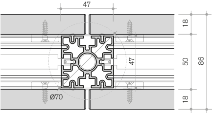
C. sezione orizzontale horizontal section
