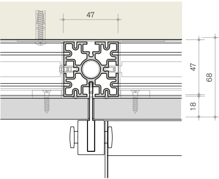
D. sezione orizzontale horizontal section
