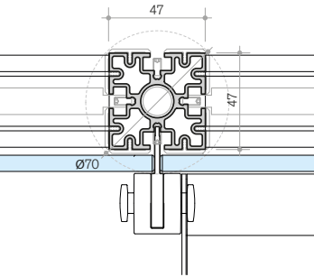
D. sezione orizzontale horizontal section
