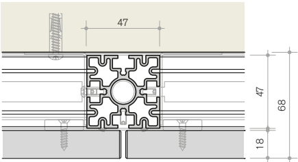
C. sezione orizzontale horizontal section
