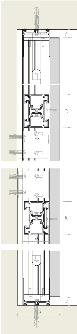
B. particolare a pavimento floor detail
