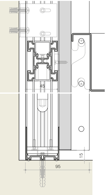
B. particolare aggancio mensola shelf hooking detail
