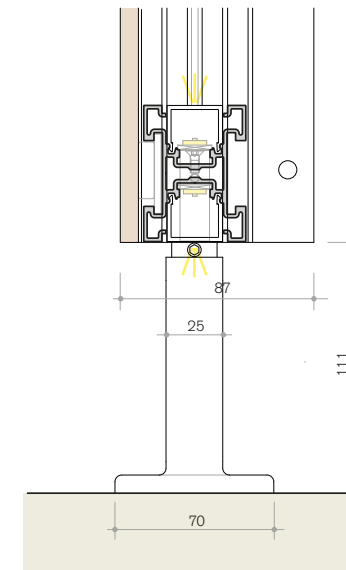
C. particolare a pavimento floor detail
