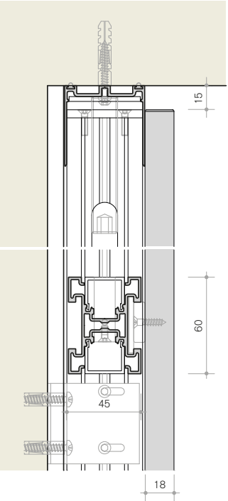
A. particolare a soffitto ceiling detail
